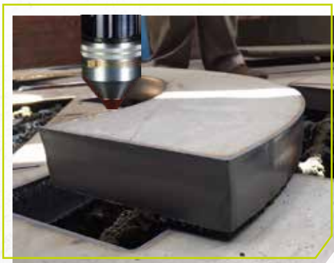
Découpe de 70 mm avec H35/N 2 à 600 A
